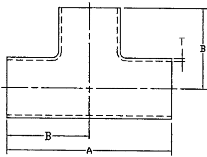
7WW 短焊三通
