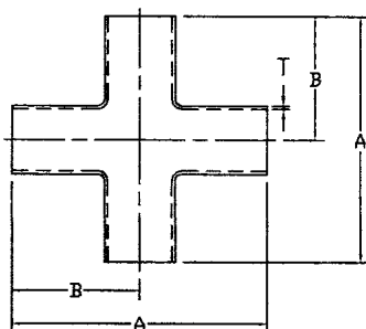
9W 長焊十字通
