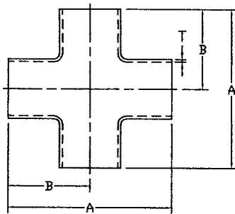
9WW 短焊十字通
