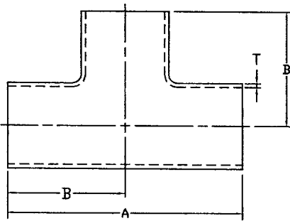
7W 長焊三通
